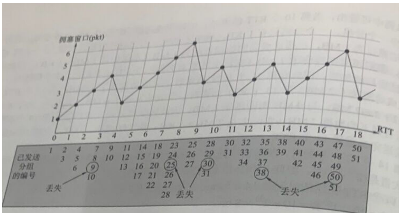
图 T-5-36 拥塞窗口与 RTT 的关系曲线
